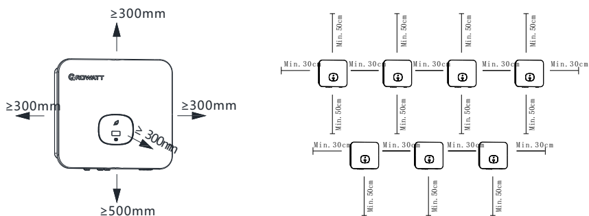
Dimensões ambientais de um inversor Dimensões ambientais de inversores em série
