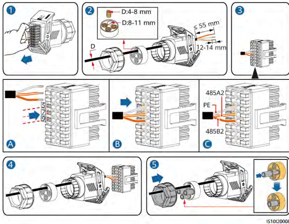
Abbildung 5-30 Kabelmontage
